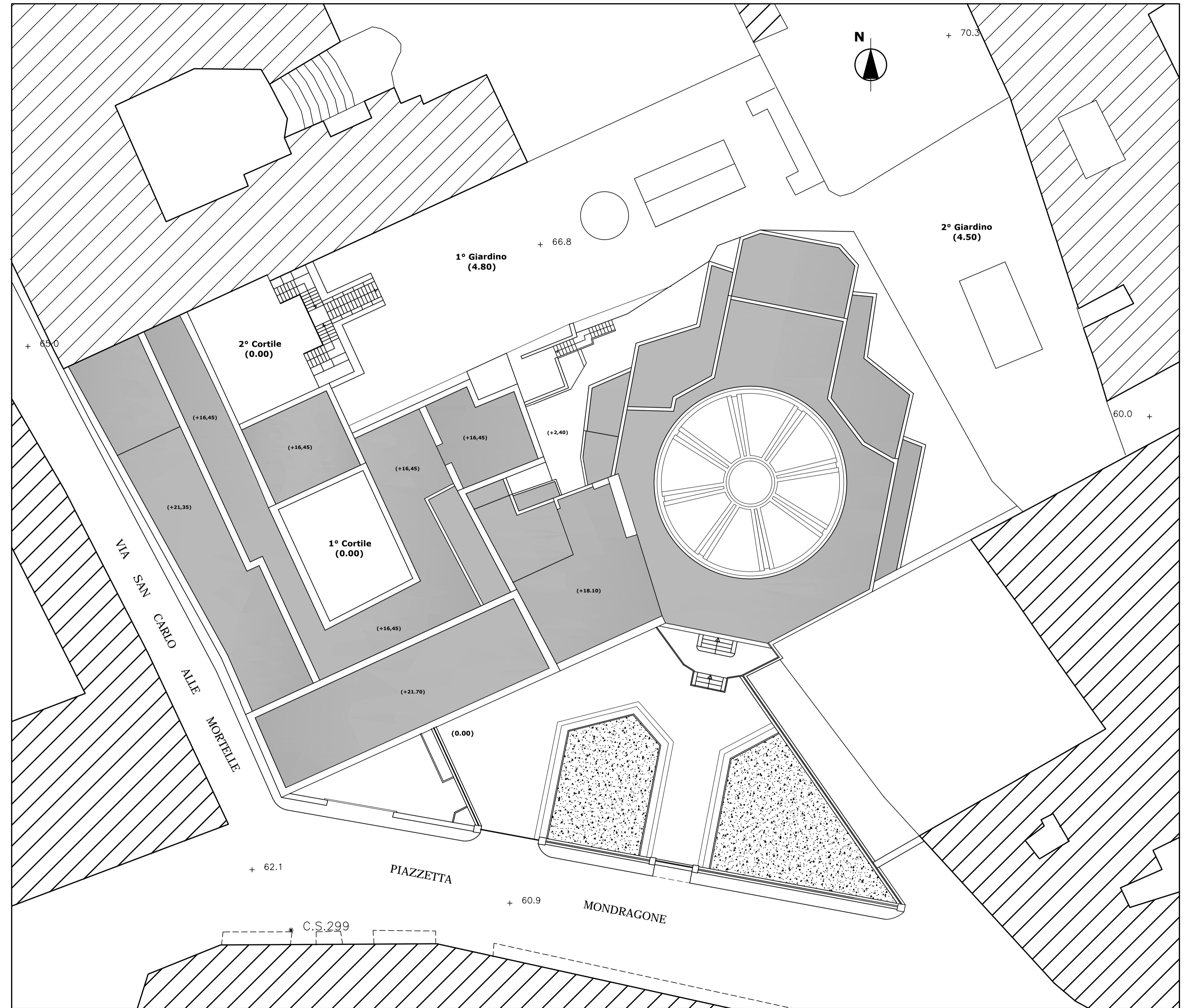
PLANIMETRIA GENERALE - RAPP.: 1/200
